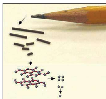
شکل (۱۰-۱): پینسل و نقاط رسم شدهٔ آن
