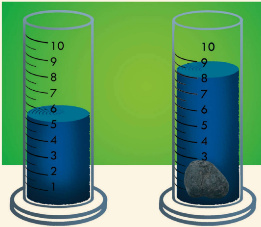
شکل (۱-۳۲) سلندر درجه دار
