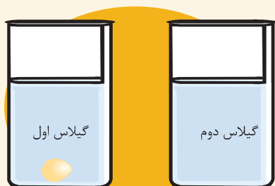
شکل (۹ - ۲) سرعت حل شدن قند خشتی در آب
