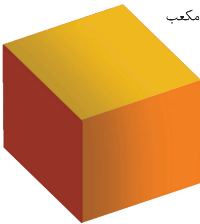
شکل (۱-۳۱) مکعب
