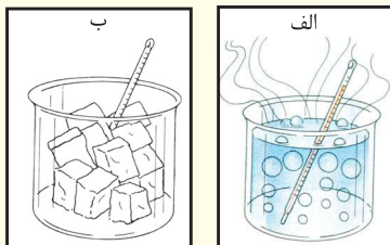
شکل (۲۰-۱) الف) انبساط سیماپ در گرما ب) انقباض سیماپ در سرما
