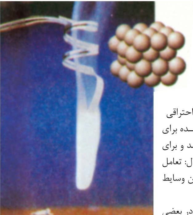
شکل (۳-۴) سوختن مگنیزیم و آزاد شدن نور و حرارت
