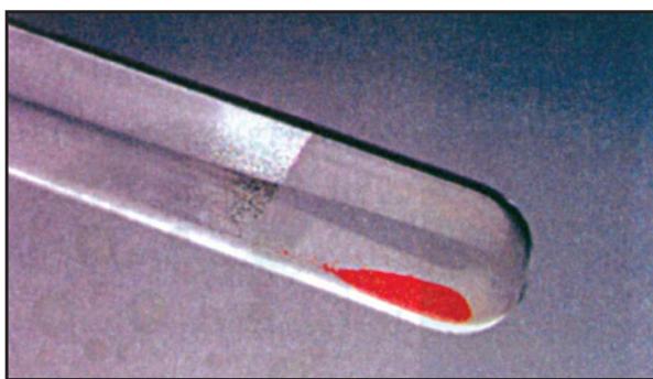
شکل (۵-۳): تجزیه اکساید سیماب
