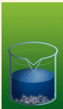
شکل (۱۰ - ۲) اثر حرارت بر حل شدن بوره در آب
