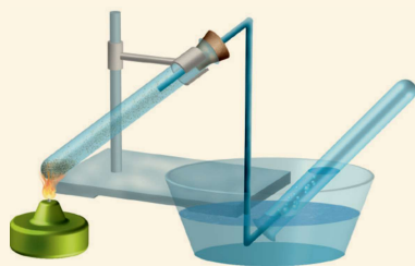
شکل (۶-۳) دستگاه تجزیه مس (II) هایدروکسی کاربونات (ملخیت)
