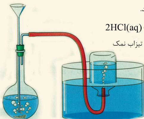
شکل (۴-۳) استحصال هایدروجن از تیزاب نمک
