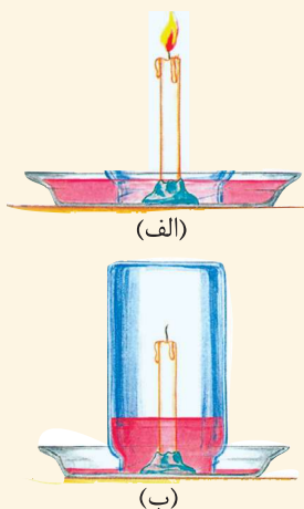
شکل (۴-۹) نقش آکسیجن در سوختن مواد
