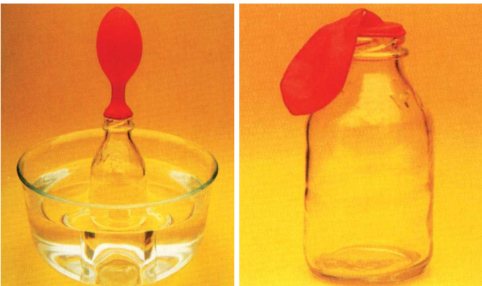
شکل (۱۹-۱) انبساط هوا در اثر حرارت
