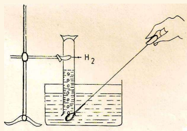
شکل (۴-۴): تعامل سدیم با آب
