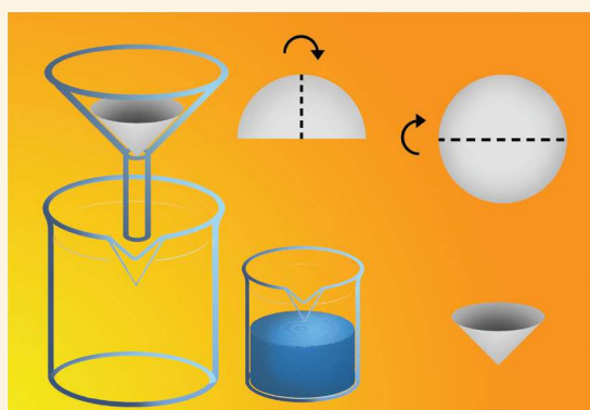
شکل (۶-۲) جدا سازی مواد توسط عملیه فلتر کردن
